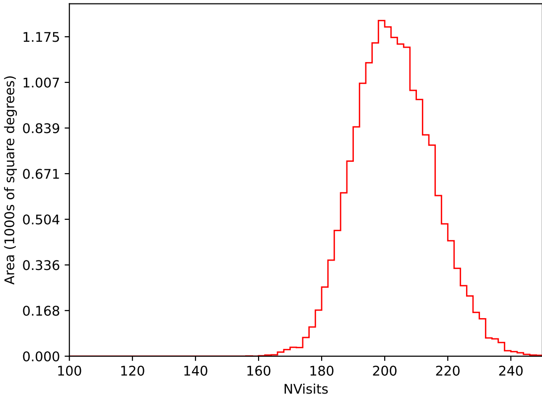
weather_cloudso4v3.4_10yrs WFD i band: NVisits
