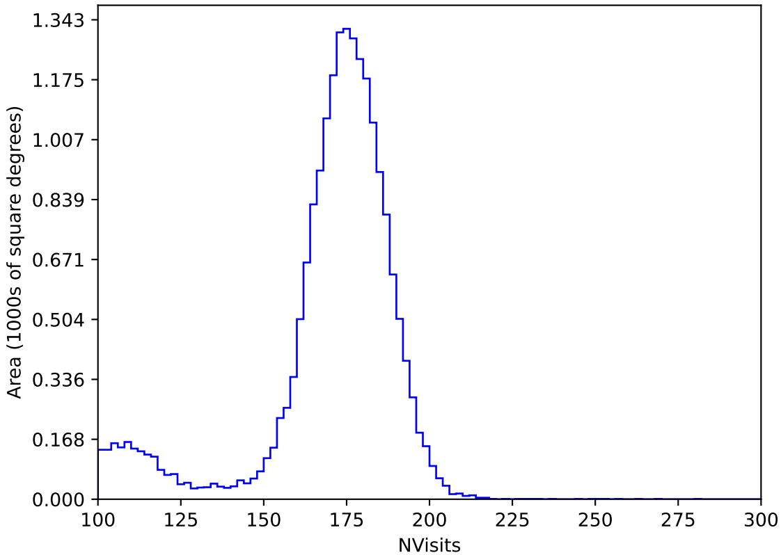
weather_cloudso4v3.4_10yrs All sky y band: NVisits
