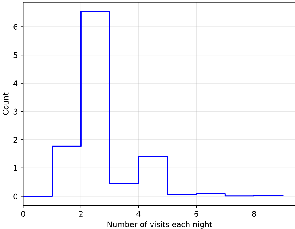
1e6 weather_cloudso4v3.4_10yrs All sky: NVisitsPerNight
