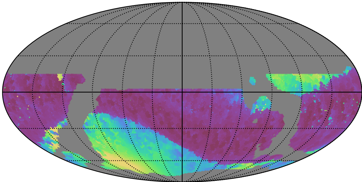
weather_cloudso4v3.4_10yrs WFD z band: Min solarElong
