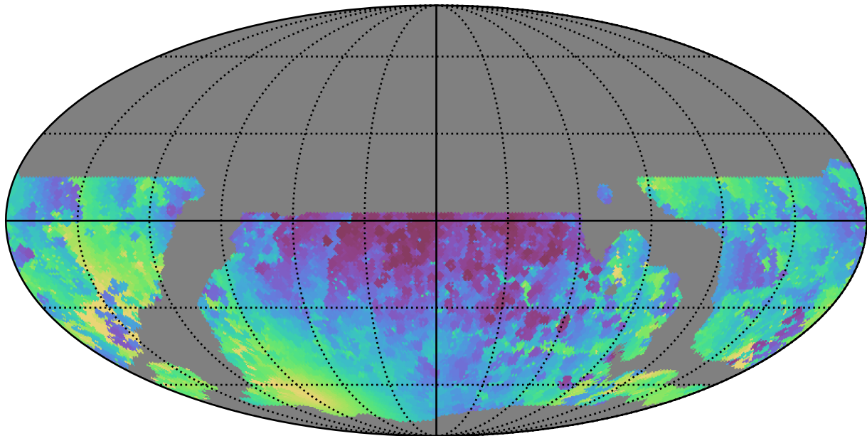
weather_cloudso4v3.4_10yrs WFD y band: Min solarElong
