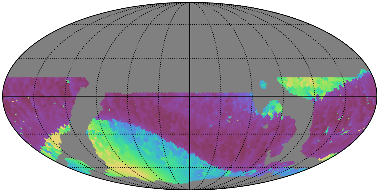
weather_cloudso4v3.4_10yrs WFD i band: Min solarElong
