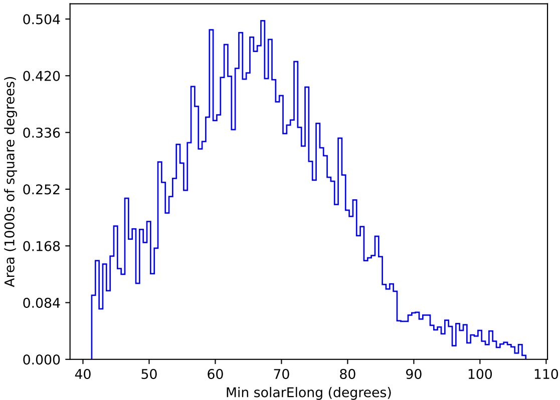
weather_cloudso4v3.4_10yrs All sky y band: Min solarElong
