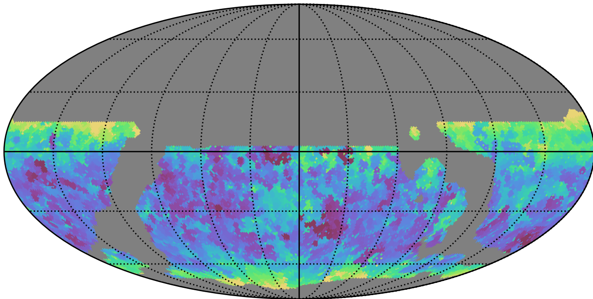
weather_cloudso4v3.4_10yrs WFD y band: Min seeingEff
