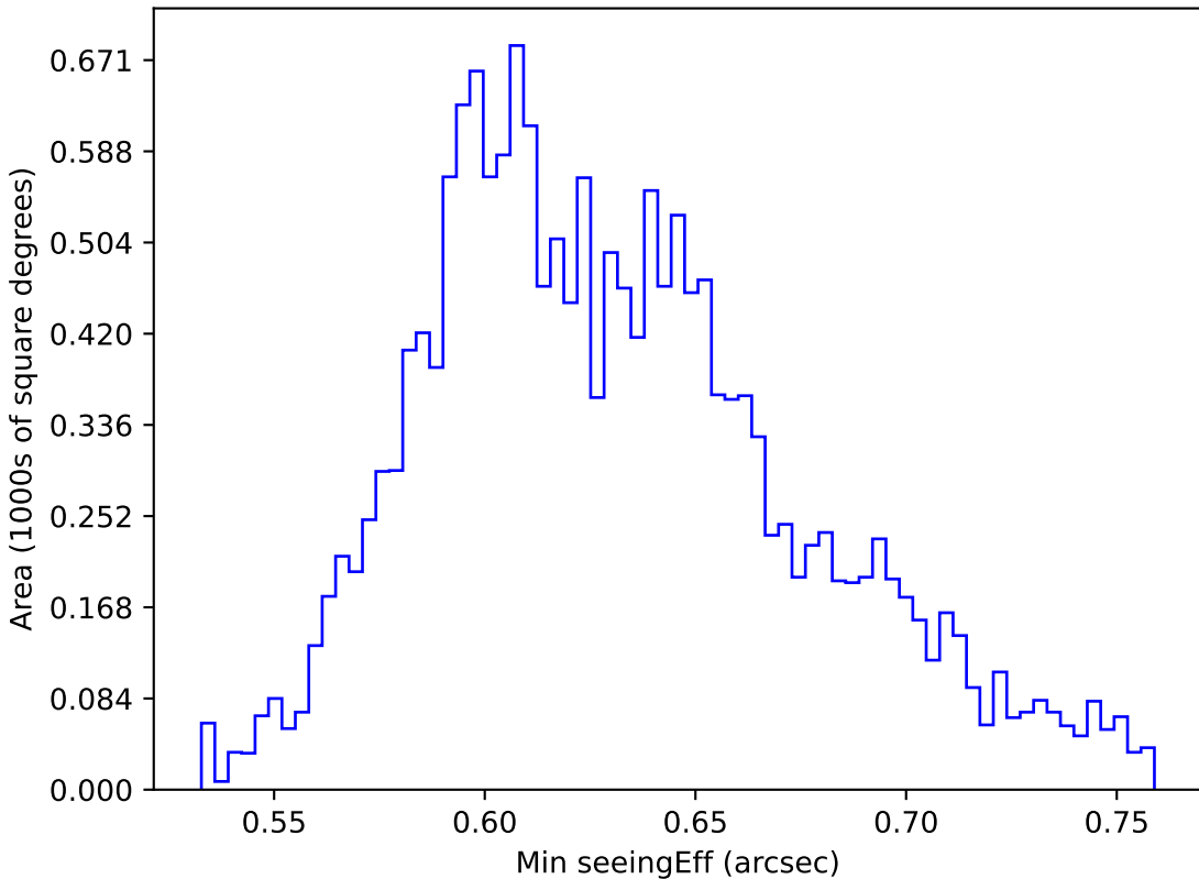
weather_cloudso4v3.4_10yrs WFD y band: Min seeingEff
