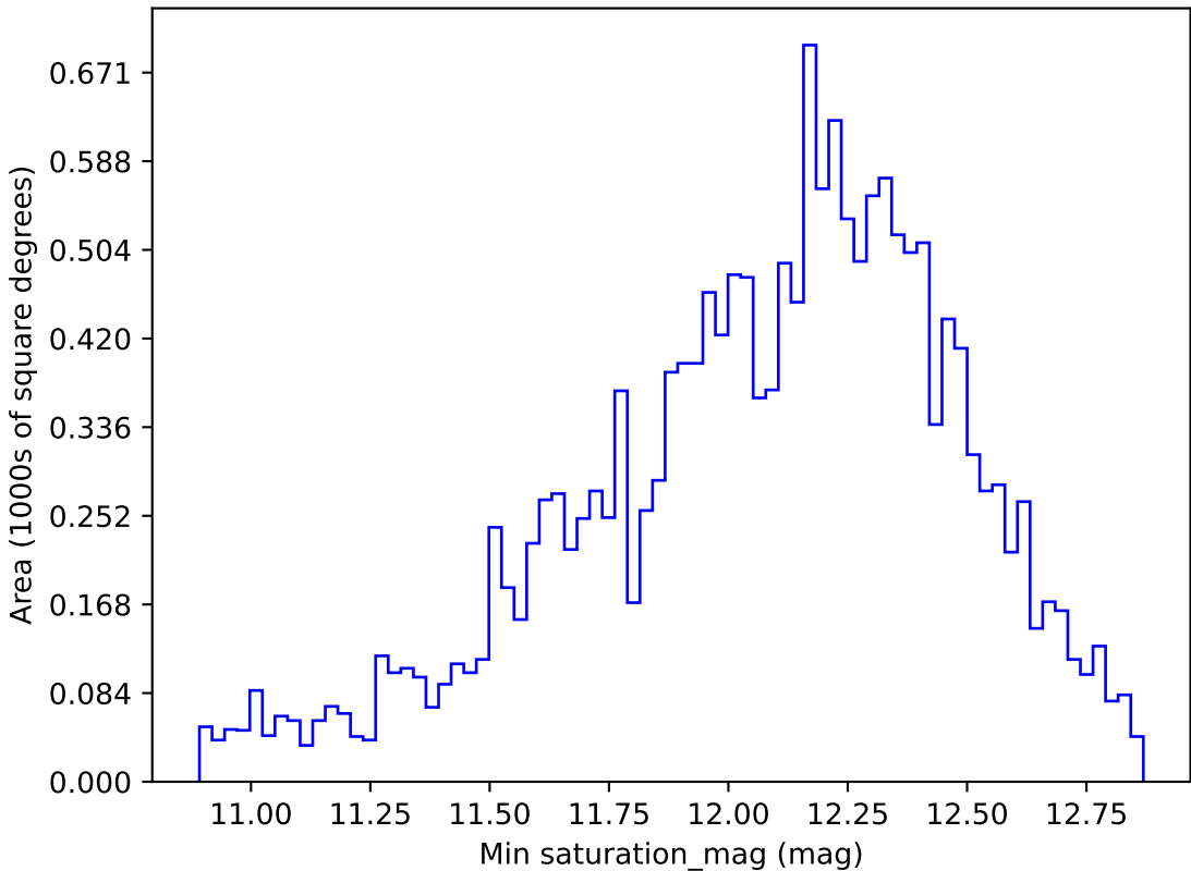
weather_cloudso4v3.4_10yrs WFD z band: Min saturation_mag
