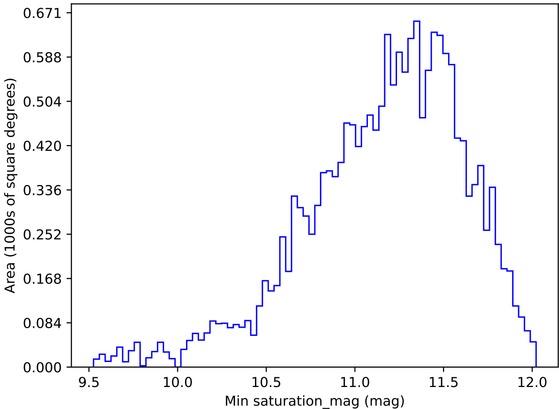
weather_cloudso4v3.4_10yrs WFD y band: Min saturation_mag
