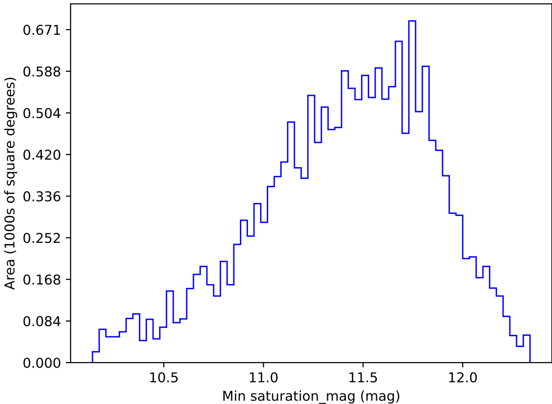
weather_cloudso4v3.4_10yrs WFD u band: Min saturation_mag
