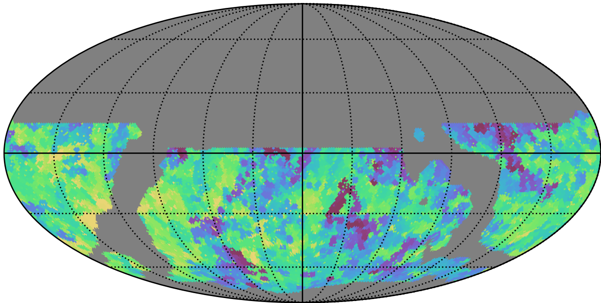
weather_cloudso4v3.4_10yrs WFD r band: Min saturation_mag
