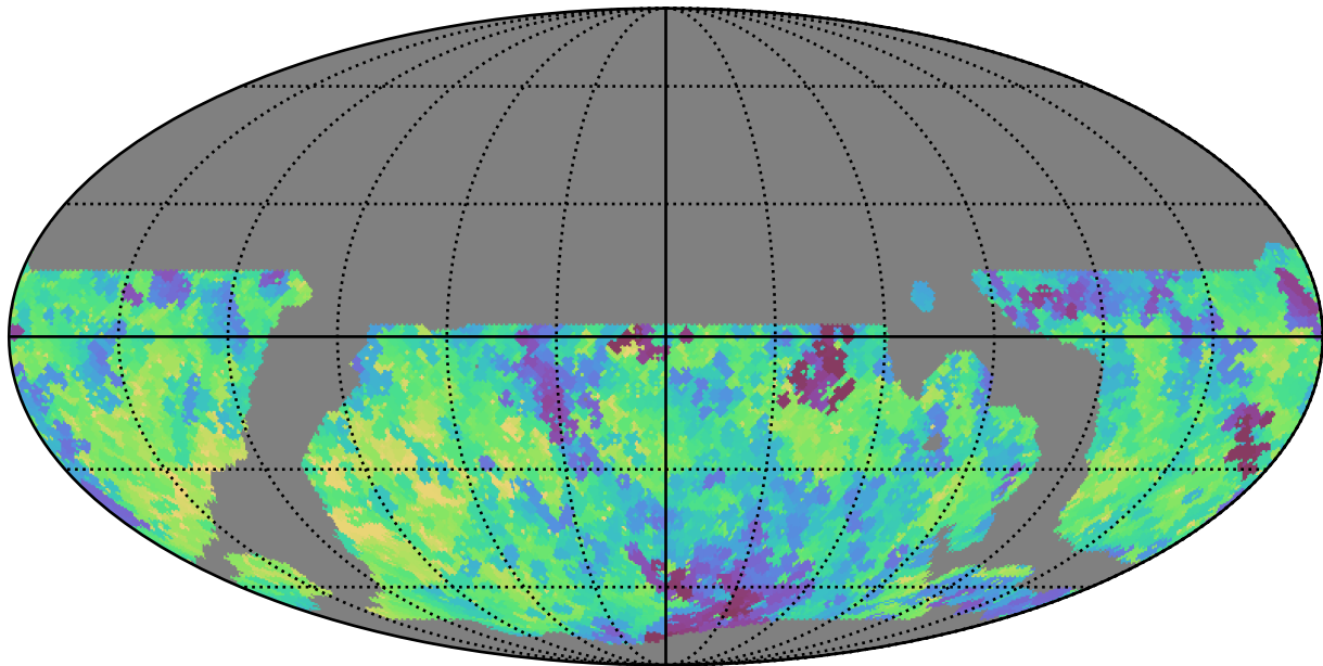
weather_cloudso4v3.4_10yrs WFD i band: Min saturation_mag
