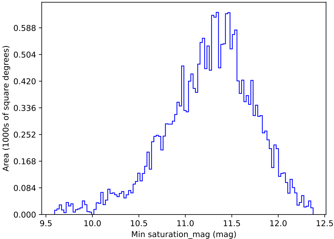
weather_cloudso4v3.4_10yrs All sky y band: Min saturation_mag
