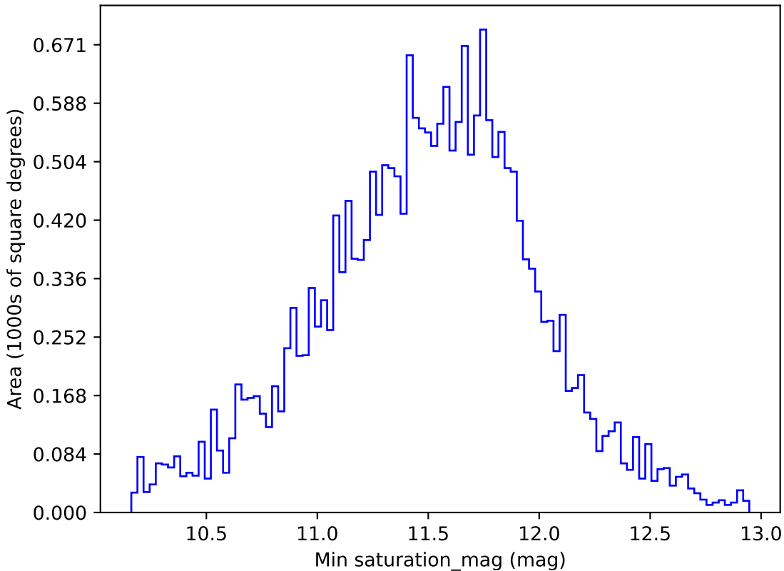
weather_cloudso4v3.4_10yrs All sky u band: Min saturation_mag
