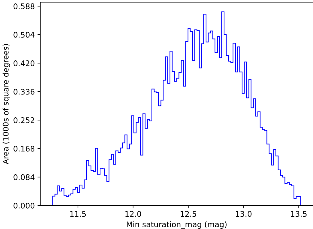
weather_cloudso4v3.4_10yrs All sky r band: Min saturation_mag
