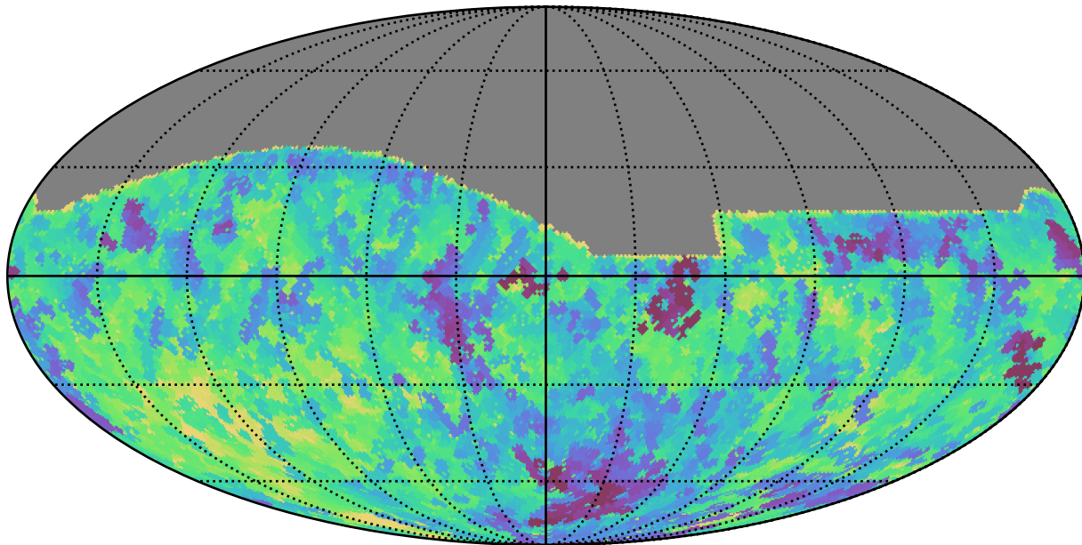
weather_cloudso4v3.4_10yrs All sky i band: Min saturation_mag
