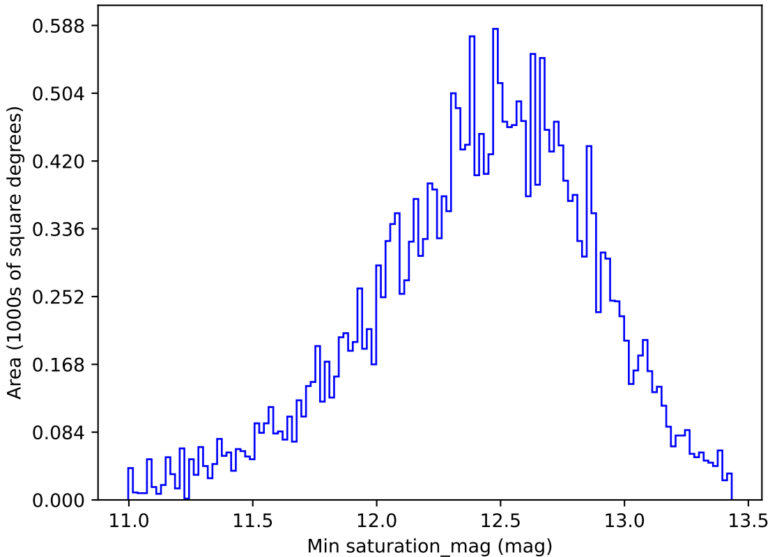
weather_cloudso4v3.4_10yrs All sky i band: Min saturation_mag
