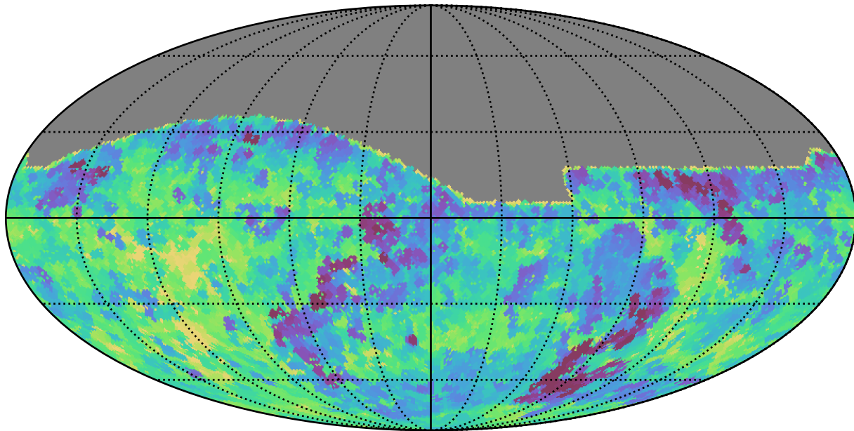
weather_cloudso4v3.4_10yrs All sky g band: Min saturation_mag
