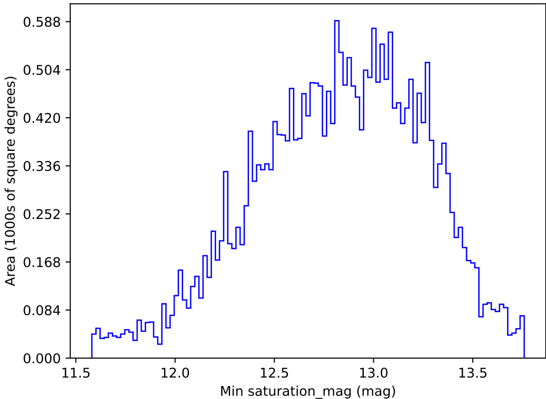
weather_cloudso4v3.4_10yrs All sky g band: Min saturation_mag
