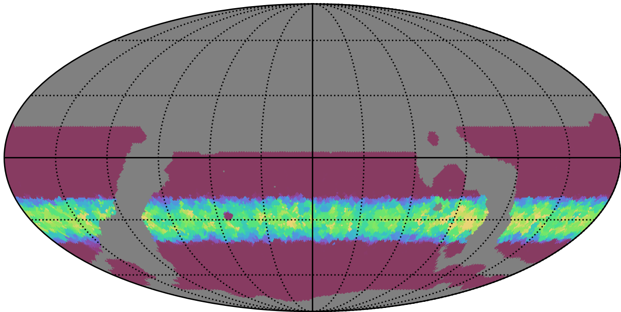
weather_cloudso4v3.4_10yrs WFD y band: Min normairmass
