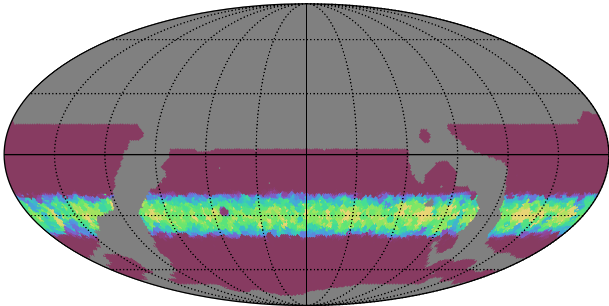
weather_cloudso4v3.4_10yrs WFD i band: Min normairmass
