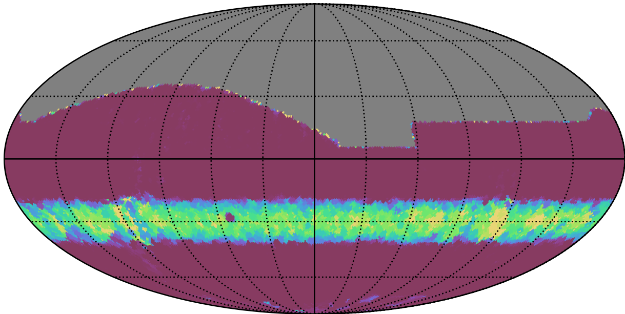
weather_cloudso4v3.4_10yrs All sky i band: Min normairmass
