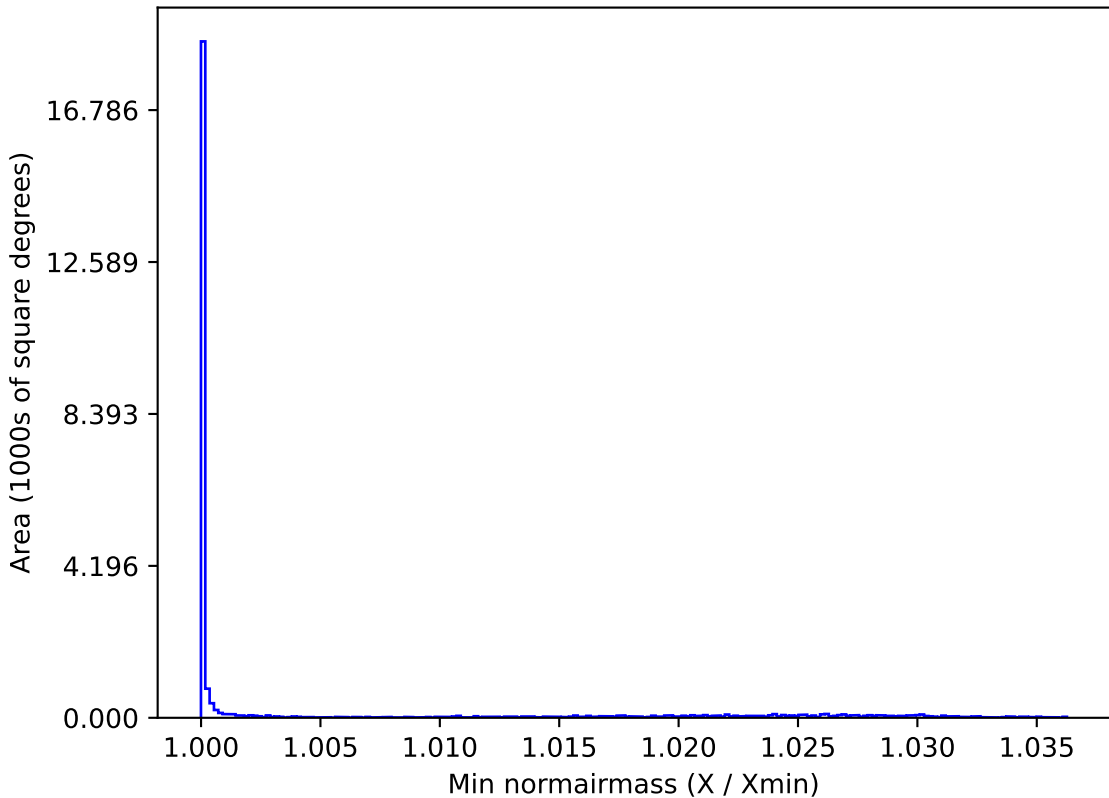
weather_cloudso4v3.4_10yrs All sky i band: Min normairmass
