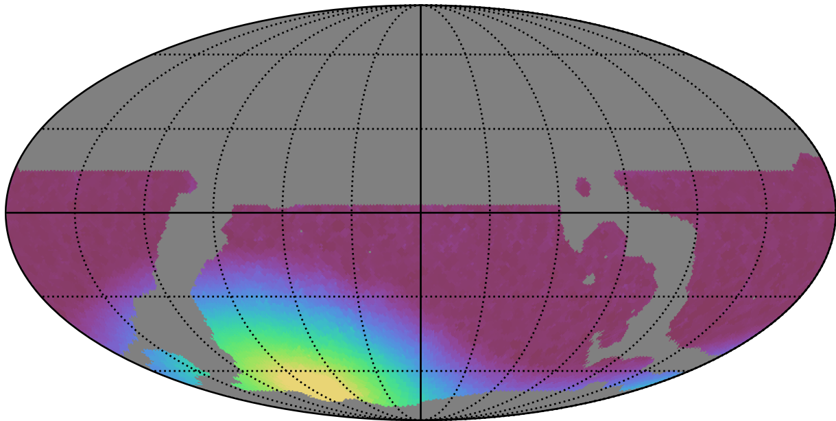
weather_cloudso4v3.4_10yrs WFD y band: Min moonDistance
