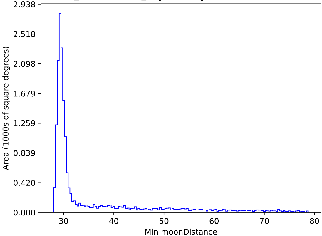
weather_cloudso4v3.4_10yrs WFD y band: Min moonDistance
