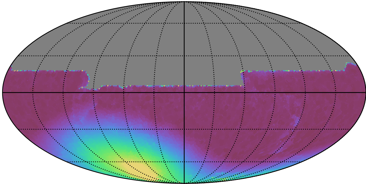
weather_cloudso4v3.4_10yrs All sky y band: Min moonDistance
