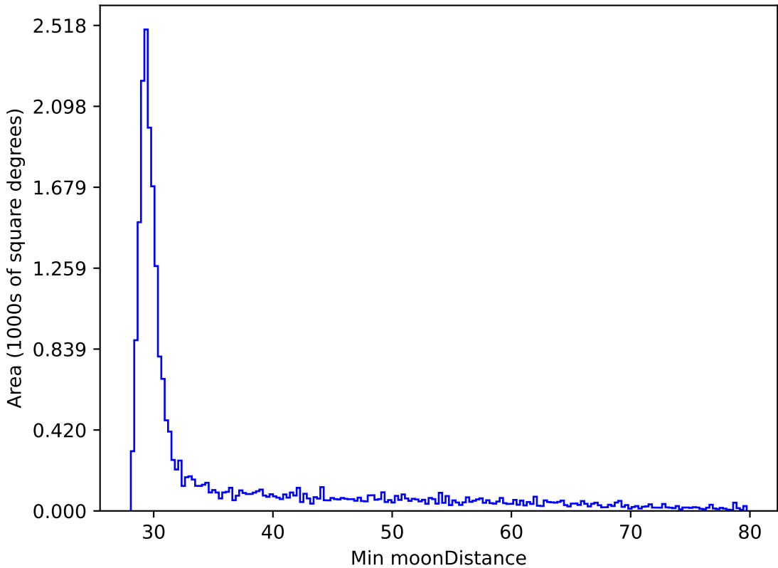
weather_cloudso4v3.4_10yrs All sky y band: Min moonDistance
