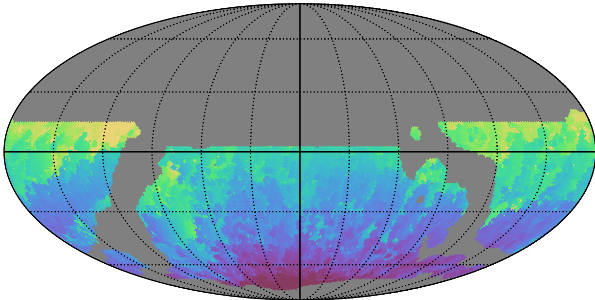
weather_cloudso4v3.4_10yrs WFD z band: Min HA
