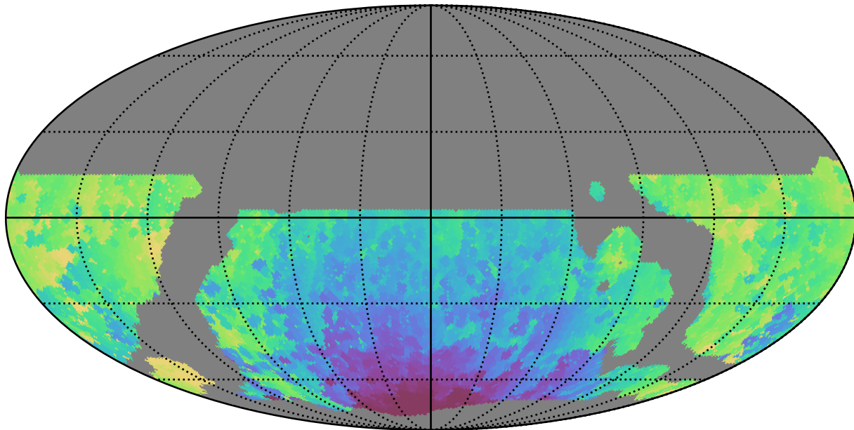
weather_cloudso4v3.4_10yrs WFD y band: Min HA
