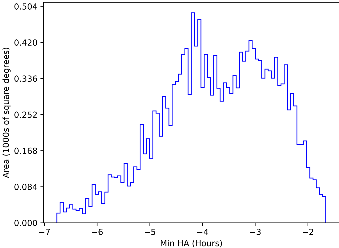
weather_cloudso4v3.4_10yrs WFD y band: Min HA
