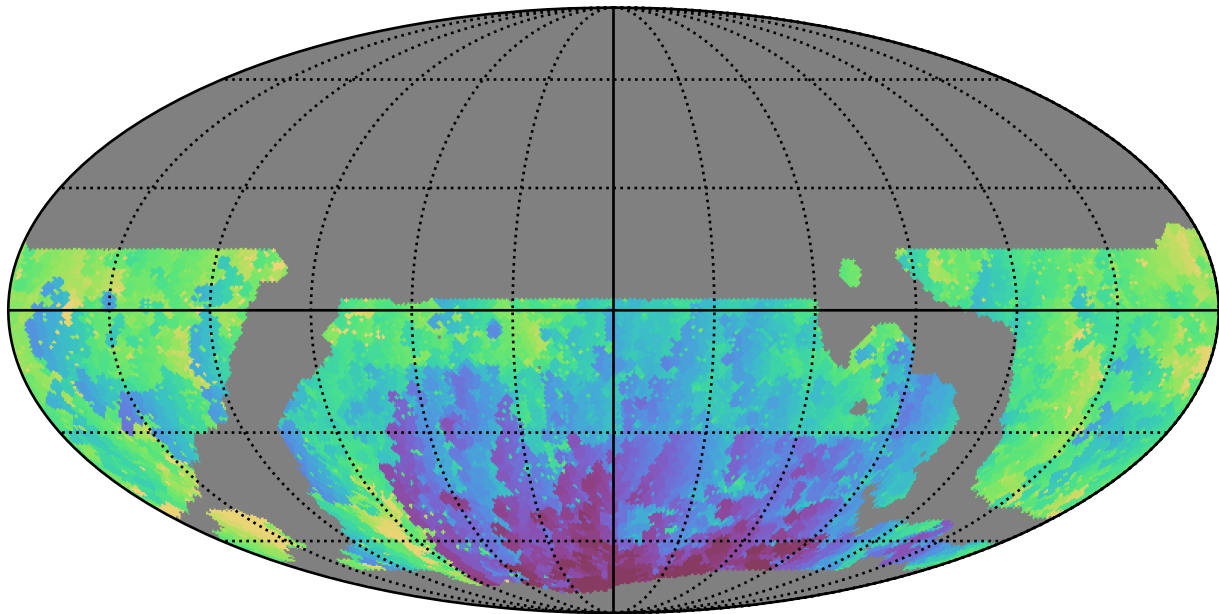
weather_cloudso4v3.4_10yrs WFD u band: Min HA
