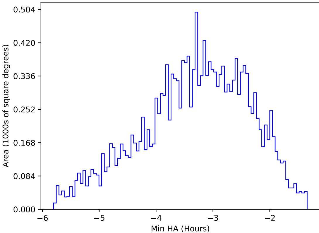
weather_cloudso4v3.4_10yrs WFD u band: Min HA
