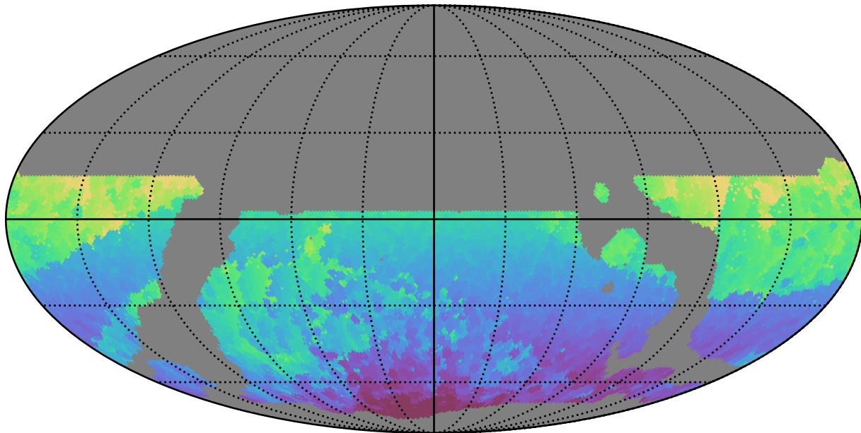
weather_cloudso4v3.4_10yrs WFD r band: Min HA
