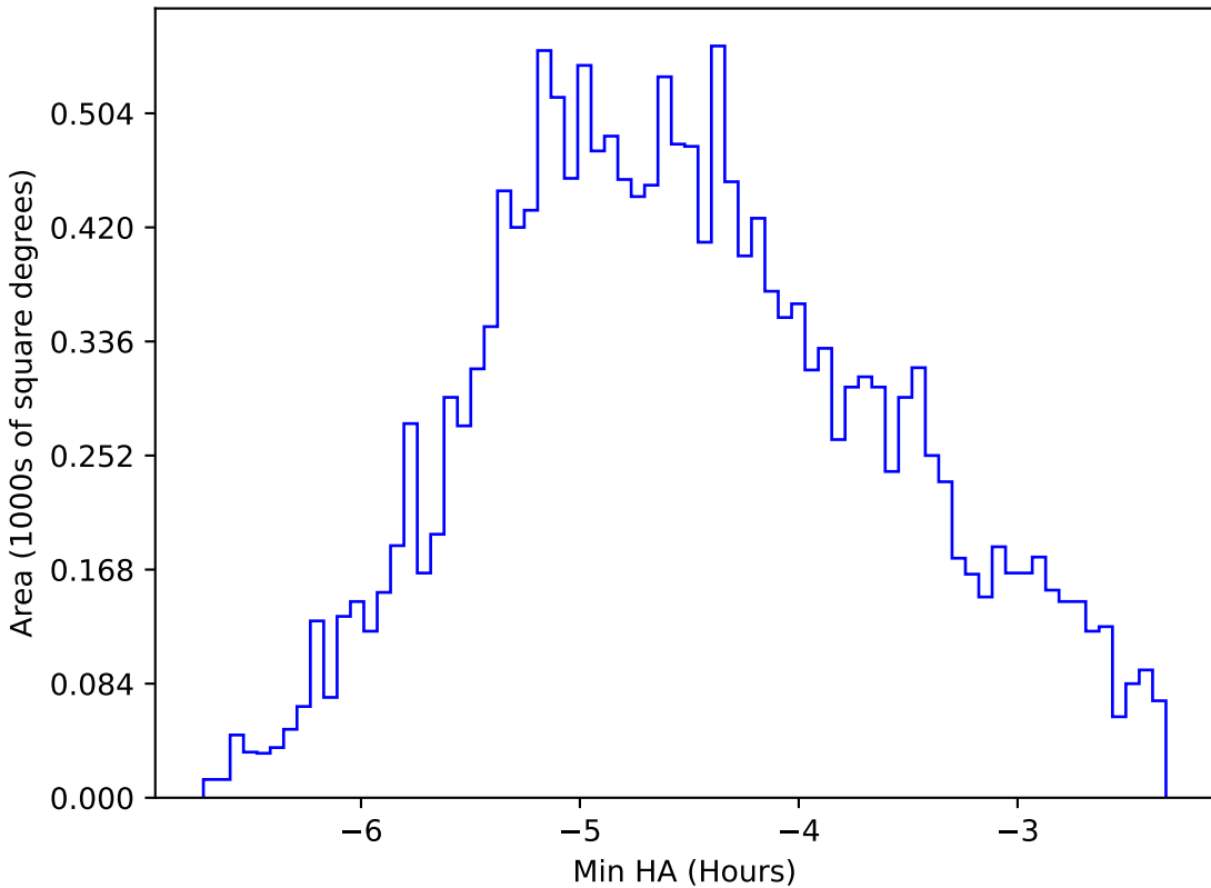
weather_cloudso4v3.4_10yrs WFD r band: Min HA
