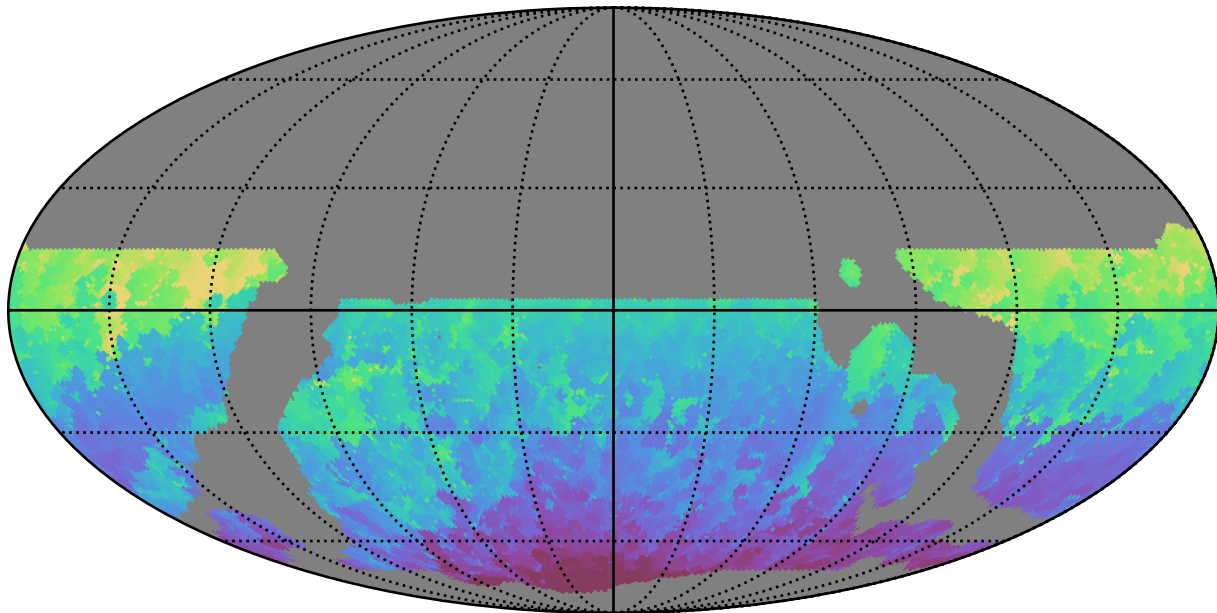
weather_cloudso4v3.4_10yrs WFD i band: Min HA
