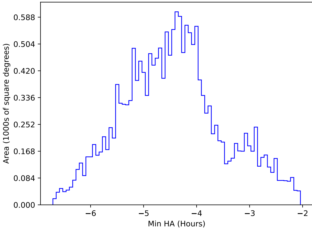
weather_cloudso4v3.4_10yrs WFD i band: Min HA
