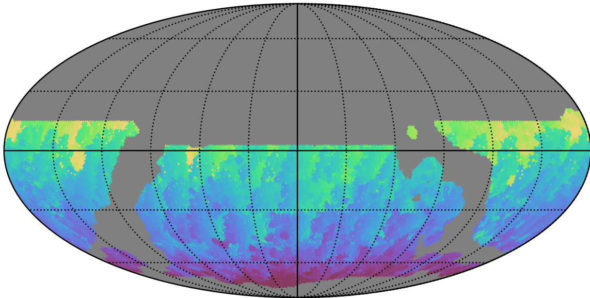
weather_cloudso4v3.4_10yrs WFD g band: Min HA
