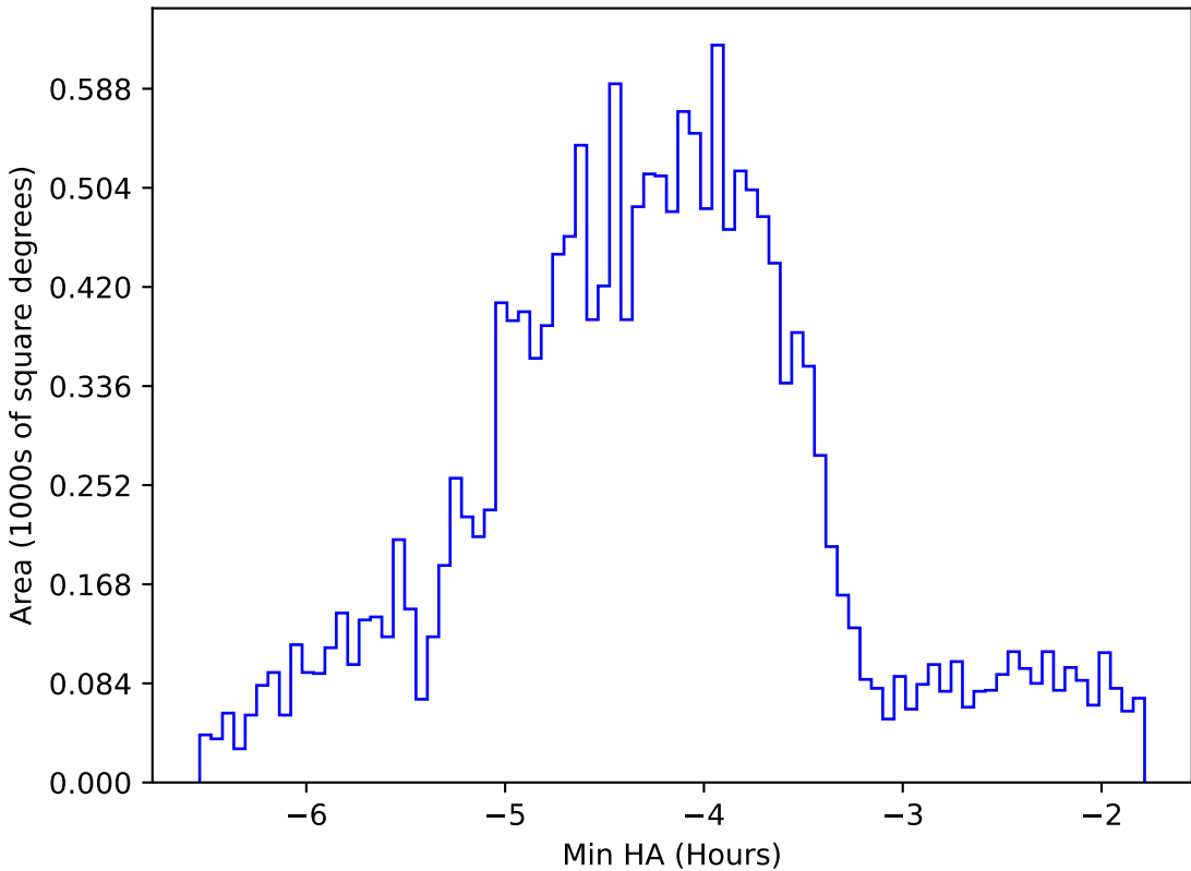
weather_cloudso4v3.4_10yrs WFD g band: Min HA
