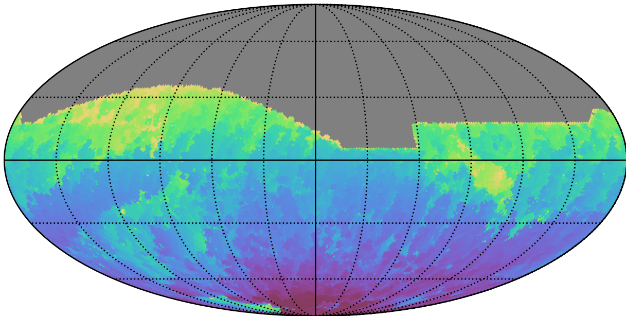
weather_cloudso4v3.4_10yrs All sky z band: Min HA
