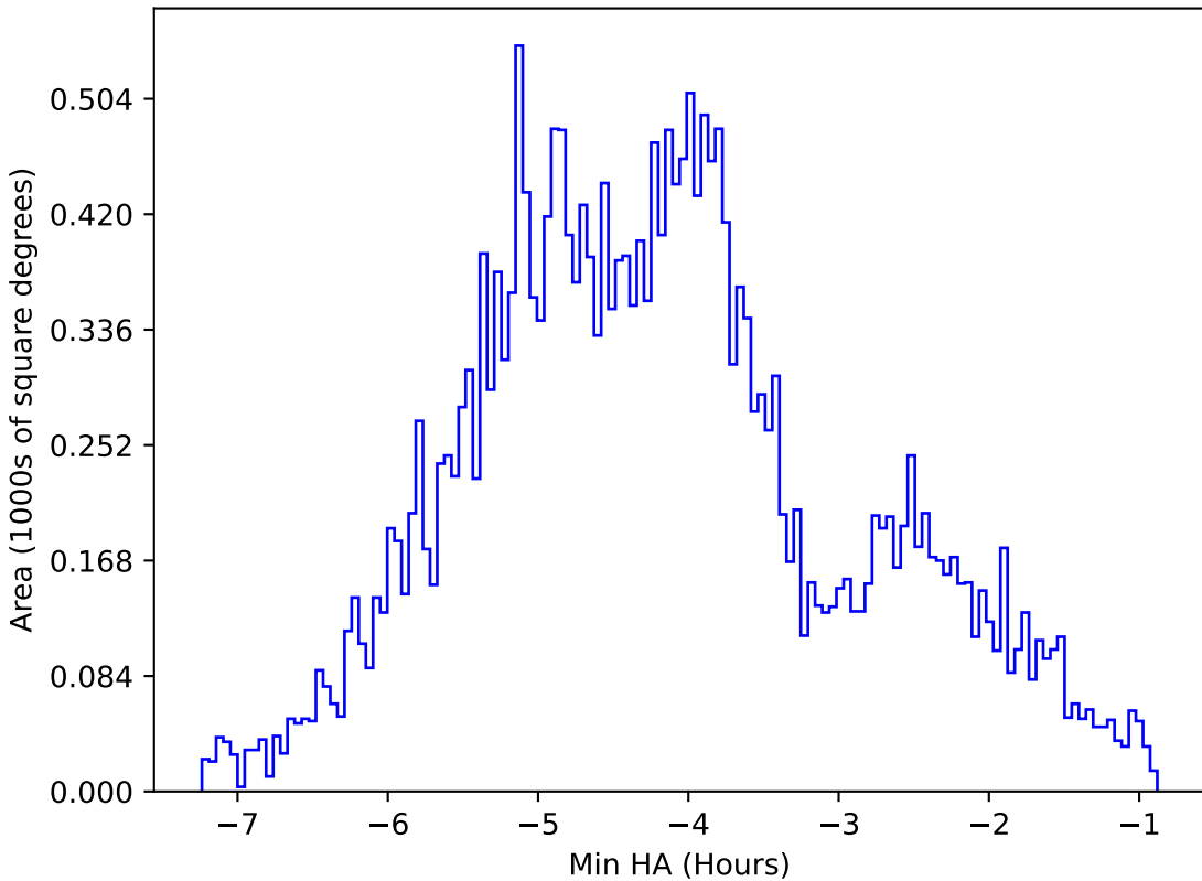
weather_cloudso4v3.4_10yrs All sky z band: Min HA
