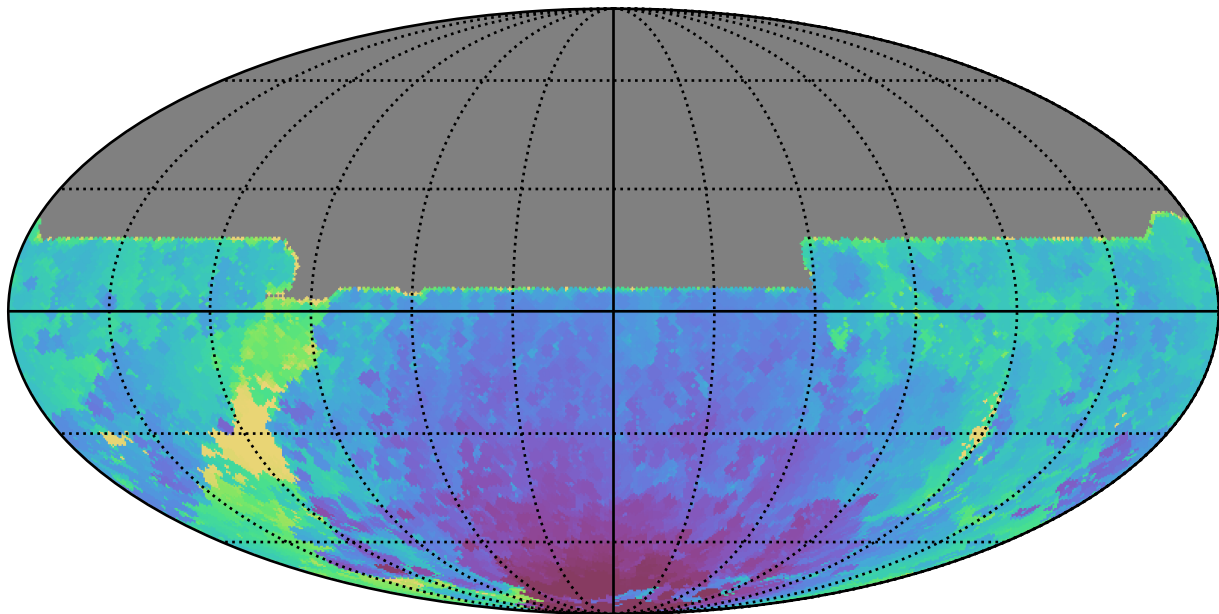
weather_cloudso4v3.4_10yrs All sky y band: Min HA
