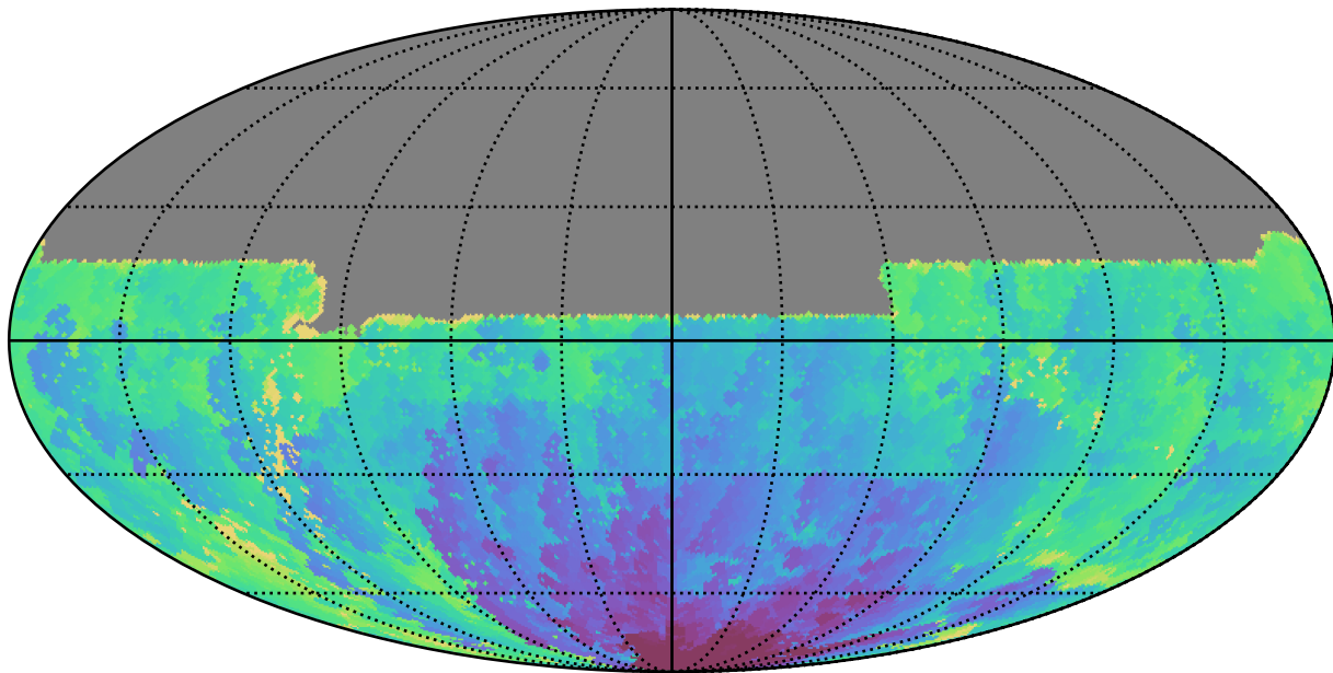
weather_cloudso4v3.4_10yrs All sky u band: Min HA
