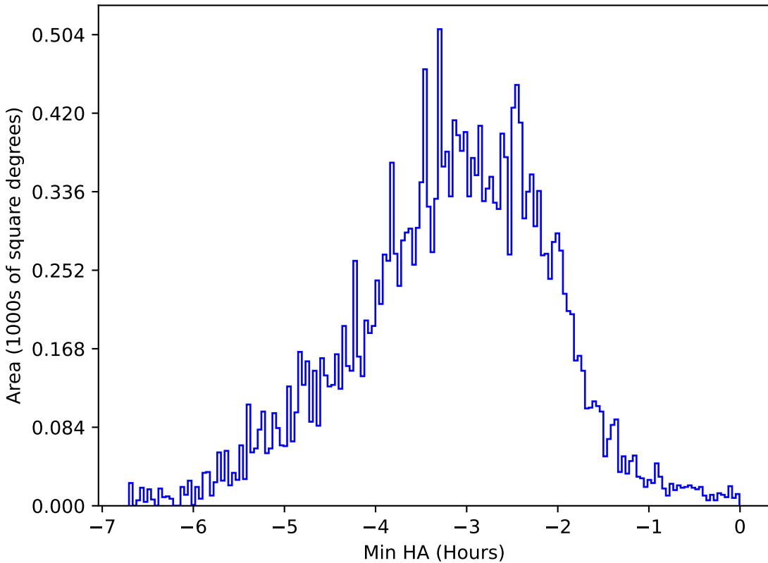
weather_cloudso4v3.4_10yrs All sky u band: Min HA
