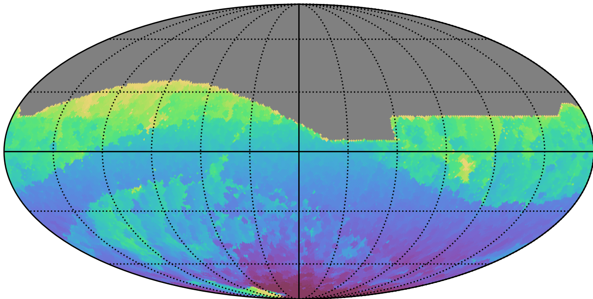
weather_cloudso4v3.4_10yrs All sky r band: Min HA
