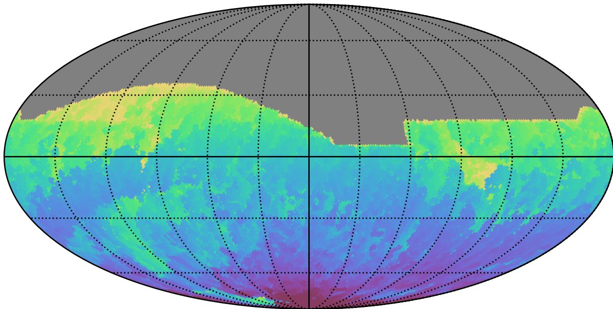
weather_cloudso4v3.4_10yrs All sky i band: Min HA
