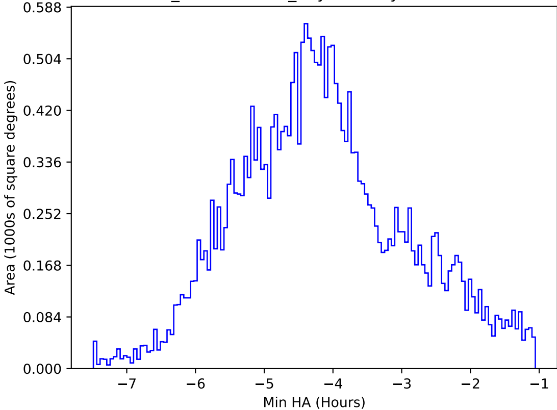
weather_cloudso4v3.4_10yrs All sky i band: Min HA
