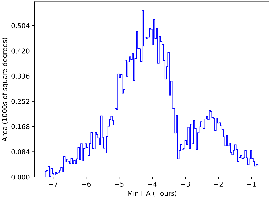
weather_cloudso4v3.4_10yrs All sky g band: Min HA
