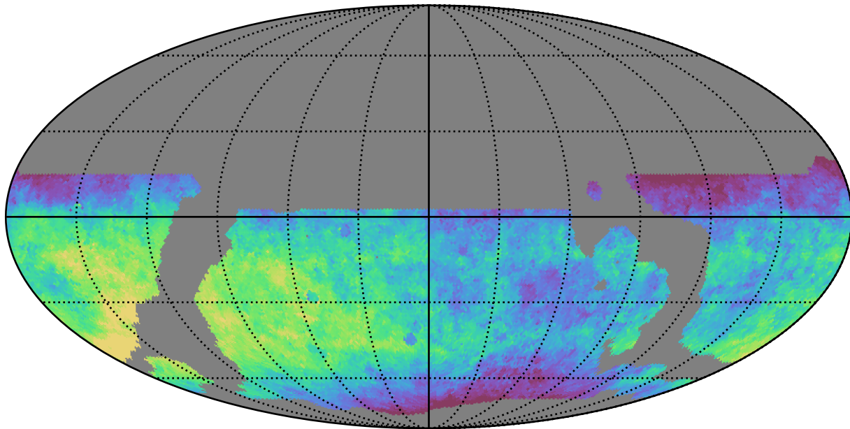
weather_cloudso4v3.4_10yrs WFD z band: Median saturation_mag
